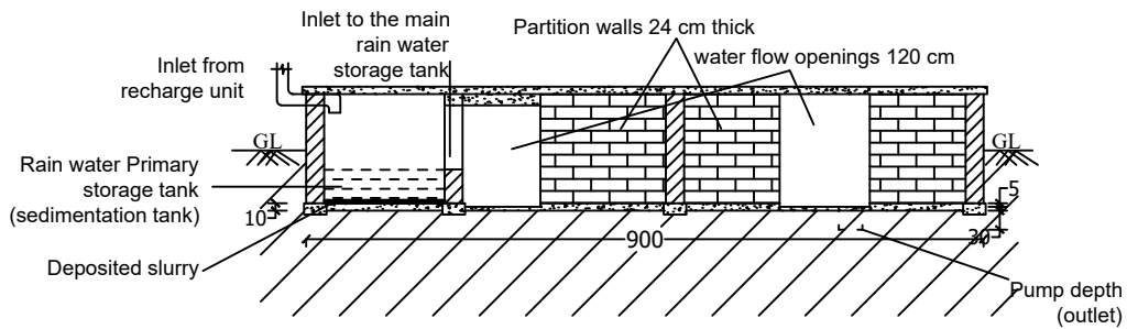
SECTION A-A
